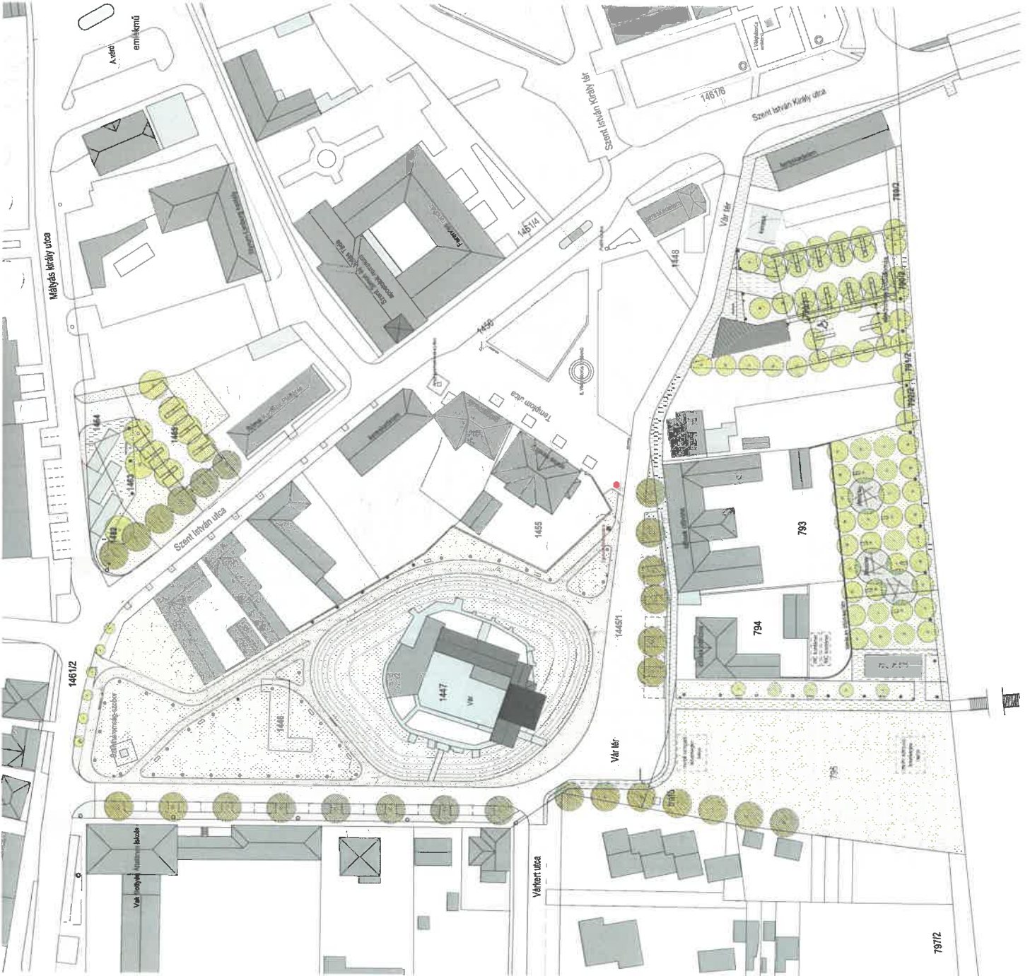
VAZRAJZ m_1:1000
