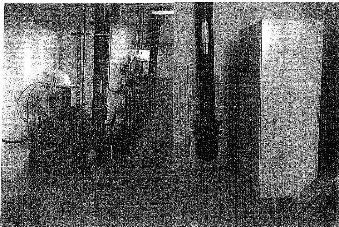
szűrőtartályok ( előtérben a homokszűrő háttérben
